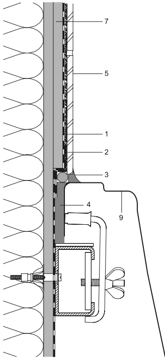
Abb. 6.4-1 Beispiel: Befestigung von Sanitäröbjekten mit Wannenleisten
