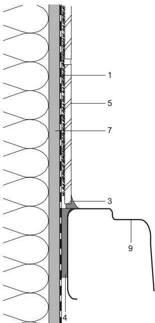
Abb. 6.4-3 Beispiel: Anschluss Duschtasse – Wand
