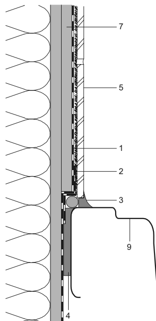
Abb. 6.4-4 Beispiel: Anschluss Duschtasse – Wand
